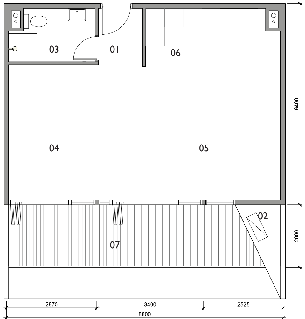
Type D1 788 sq.ft (73 sq.m)
